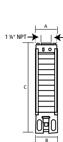
Acoplamiento NEMA 4"
